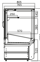
VVSTPD - VD padaria bakery boulangerie panadería
