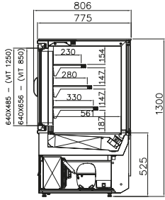
VVSTGL - VD 3L1 sobremesas geladas frozen desserts entremets glacés postres helados
