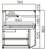
CXEVST - VD caixa expositora exposition case caisse d'exposition caja expositora
