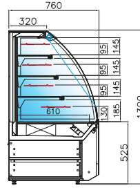
VMVSTVS - VS 3M2 grab'n'go grab'n'go ventilée grab'n'go avec portes côté de service grab'n'go
