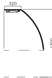
OPÇÃO: VC vidro frontal curvo curved frontal glass vitrage convexe vidrio curvo
