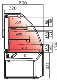
VVSTAQ - VS (***) grab'n'go aquecido c/ portas heated grab'n'go w/ rear service doors chaudé grab'n'go avec portes côté de service grab'n'go caliente c/ puertas traseras
