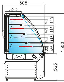
VVSTVS - VS 3M2 (*) ventilada grab'n'go c/ portas ventilated grab'n'go w/ rear service doors ventilée grab'n'go avec portes côté de service ventilada grab'n'go c/ puertas traseras
